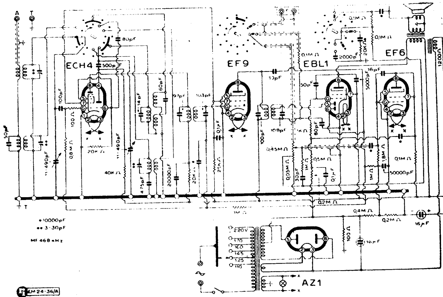
PHILIPS RADIO - MODD, « BI 480/A » « BI 481/A »
